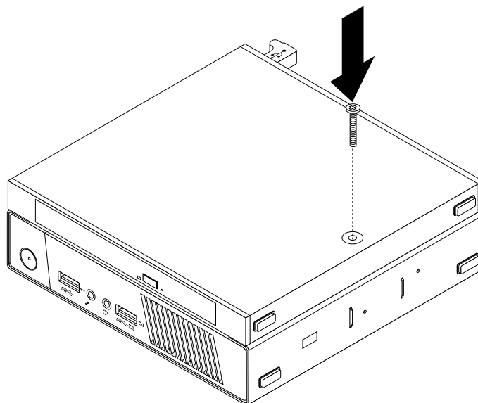
Figure 22. Installation de la vis de fixation du coffret du disque optique
