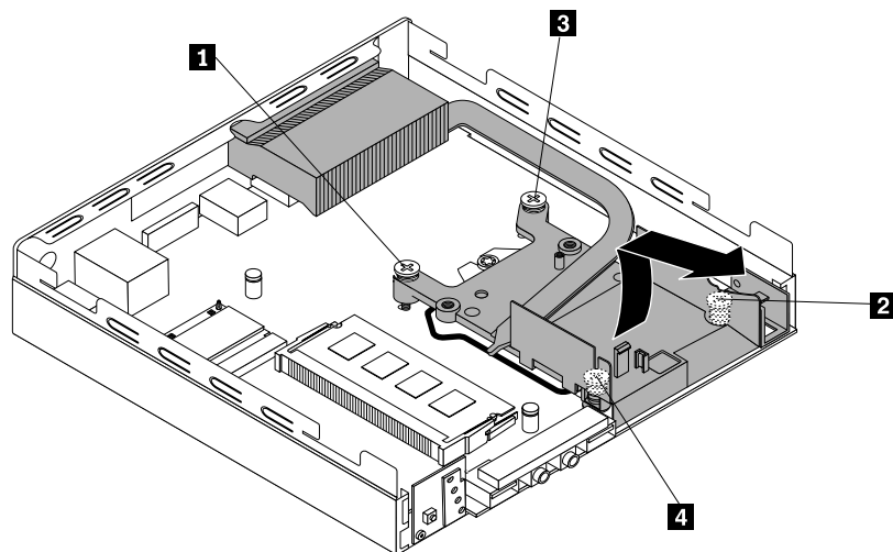
Figure 68. Retrait du module thermique
