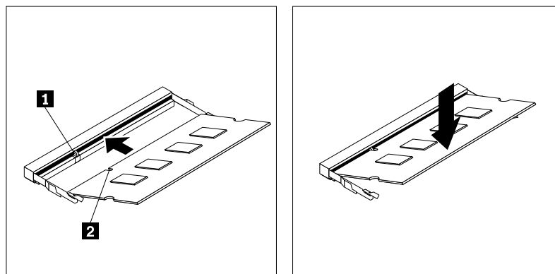
Figure 44. Installation d'un module de mémoire
