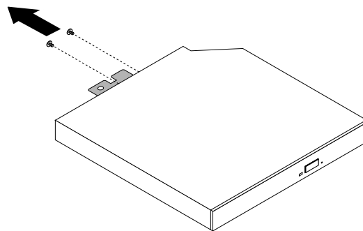
Figure 17. Retrait de la plaque métallique du disque optique
