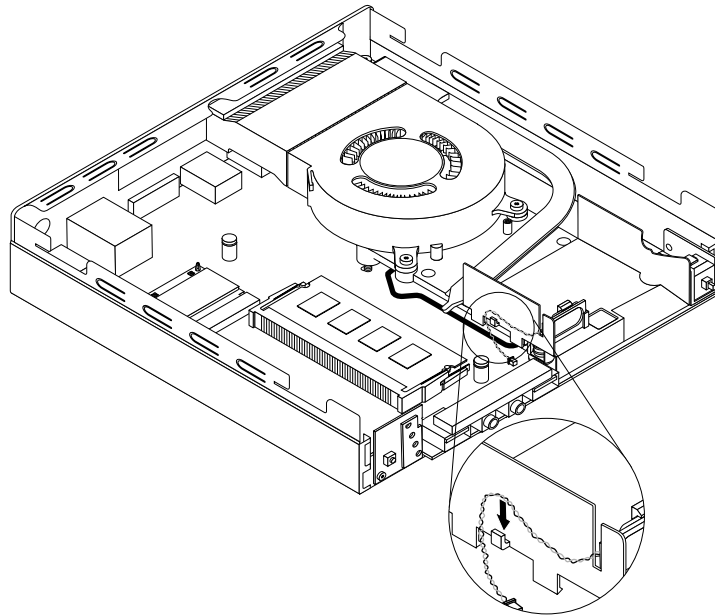
Figure 63. Fixation du câble du haut-parleur interne
