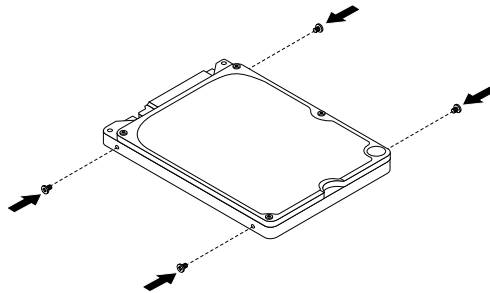
Figure 27. Installation des vis sur l'unité de disque dur
