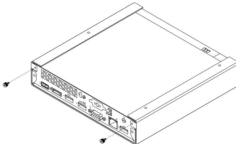
Figure 13. Retrait des vis de fixation du support de montage VESA
