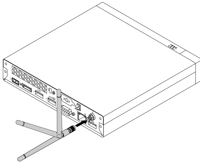
Figure 58. Installation de l'antenne Wi-Fi arrière
