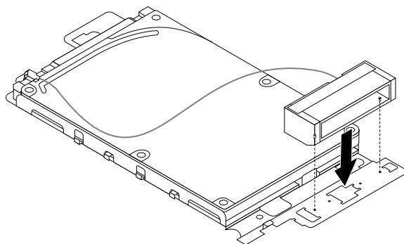
Figure 54. Fixation de l'antenne Wi-Fi avant
