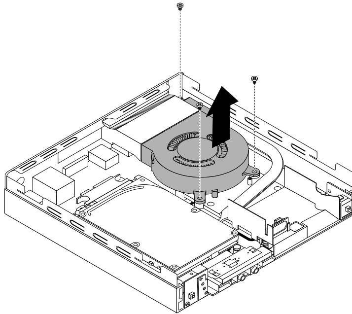
Figure 66. Retrait du ventilateur système
