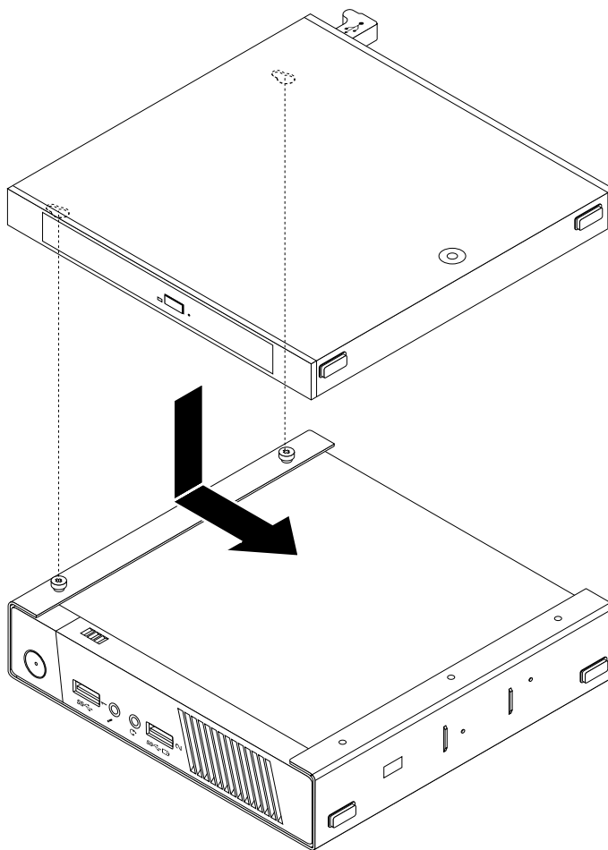
Figure 21. Installation du coffret du disque optique
