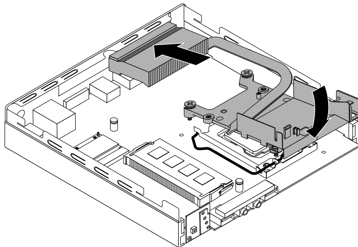
Figure 69. Installation du module thermique
