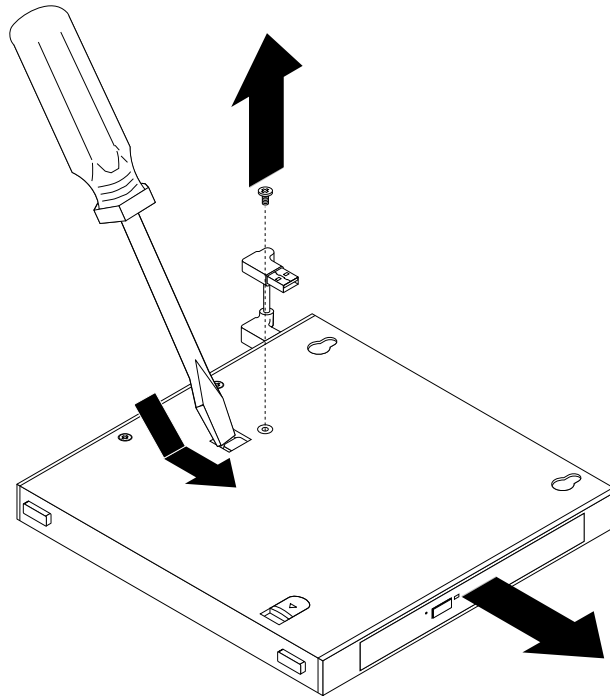
Figure 16. Retrait du disque optique de son coffret
