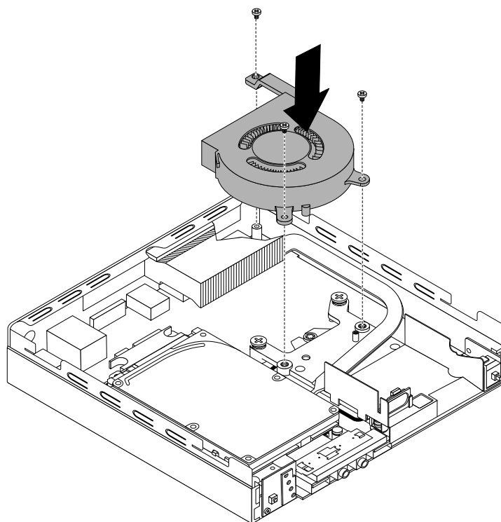
Figure 67. Installation du ventilateur système
