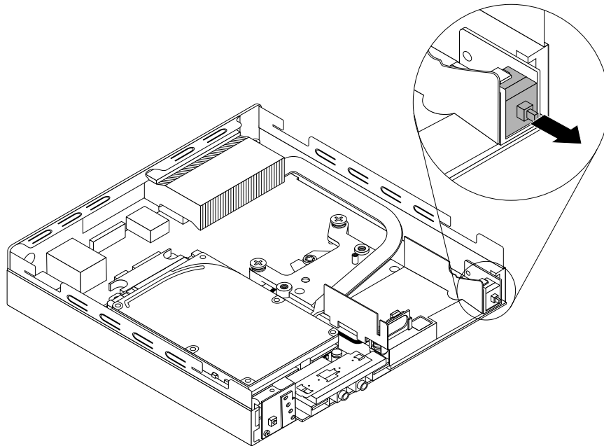
Figure 64. Retrait de l'interrupteur de détection de présence du carter
