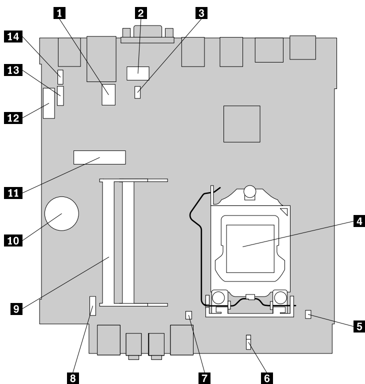
Figure 4. Emplacements des composants sur la carte mère
