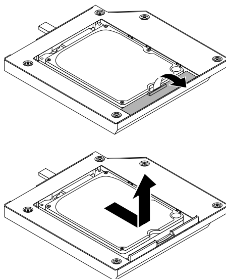
Figure 26. Retrait de l'unité de disque dur secondaire du système de retenue
