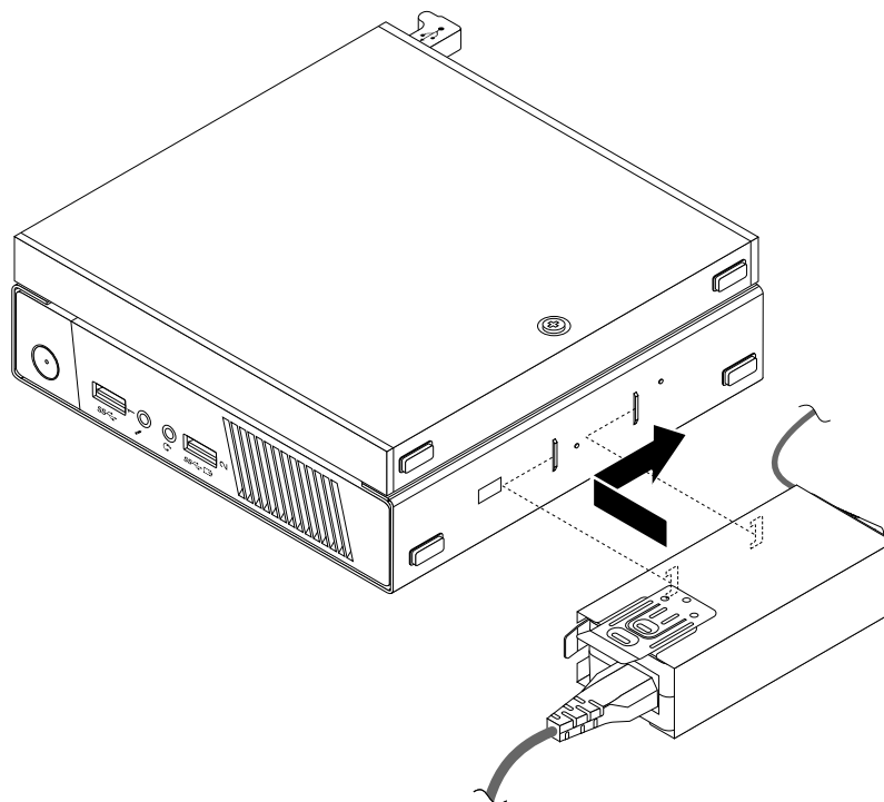
Figure 37. Installation du système de retenue du boîtier d'alimentation
