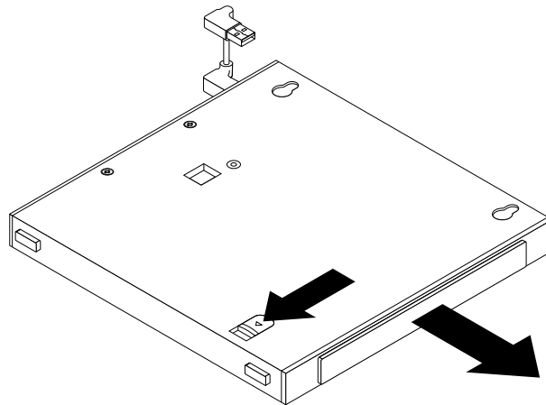
Figure 24. Retrait de la carte de l'unité de disque dur secondaire dans le coffret du disque optique
