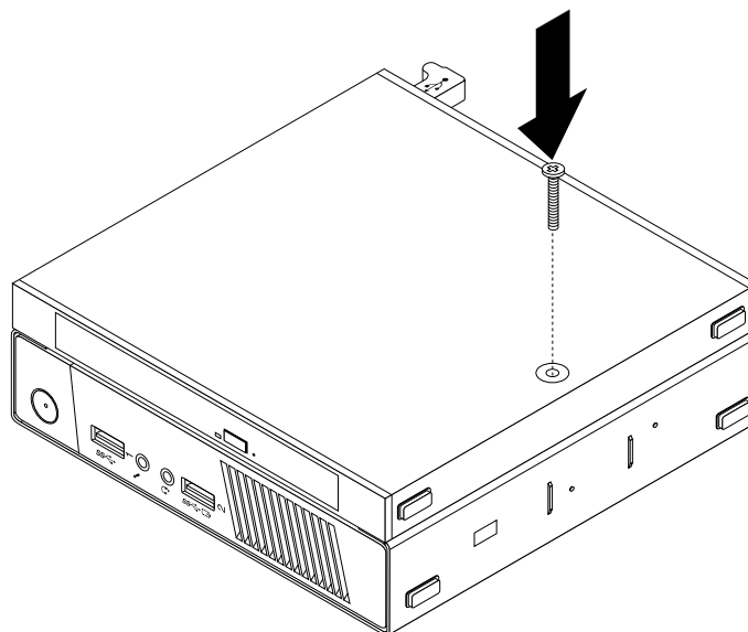
Figure 32. Installation de la vis de fixation du coffret du disque optique
