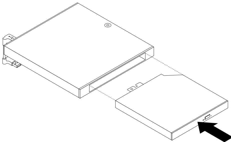
Figure 19. Installation du disque optique dans son coffret
