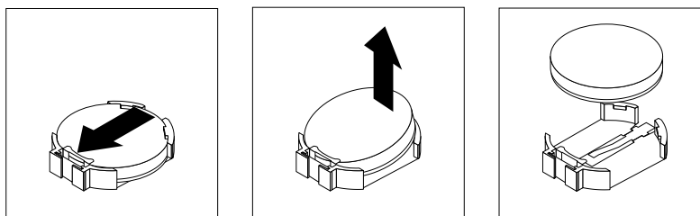
Figure 45. Retrait de l'ancienne pile
