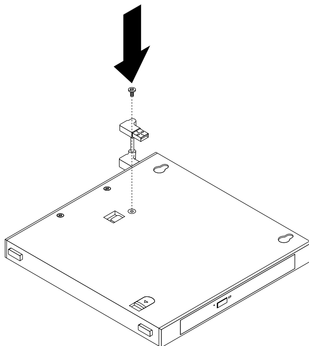
Figure 20. Installation de la vis de fixation du disque optique
