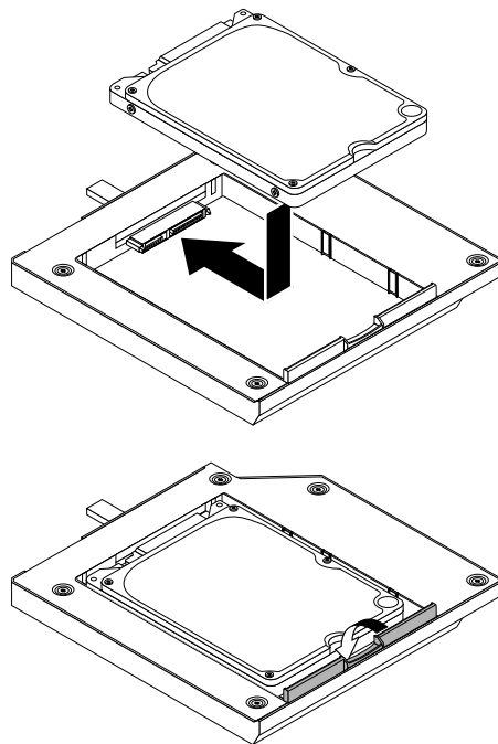
Figure 28. Installation de l'unité de disque dur dans le système de retenue
