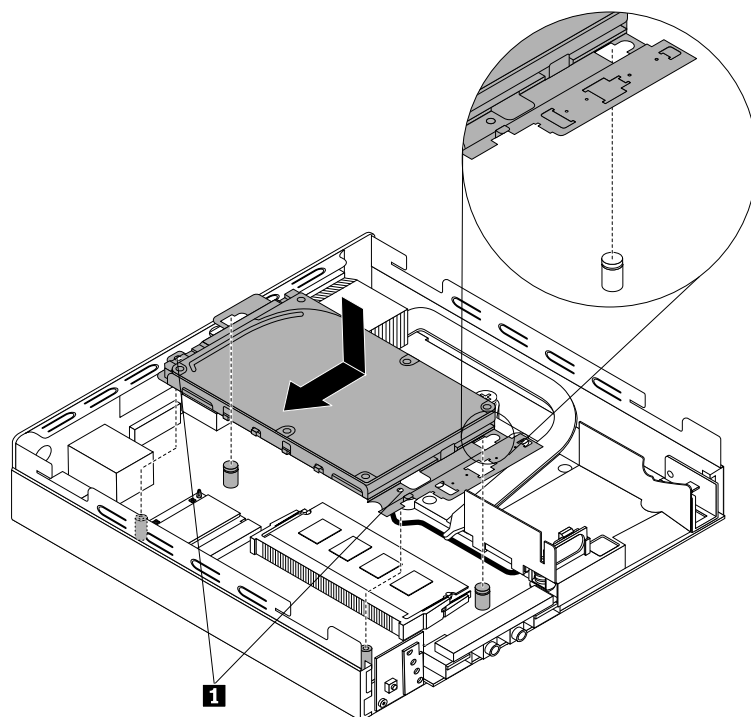
Figure 41. Installation de l'unité de disque dur
