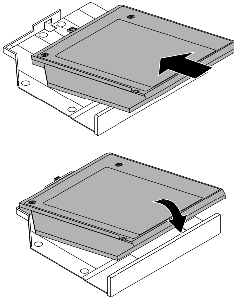
Figure 29. Installation de la carte de l'unité de disque dur dans le système de retenue
