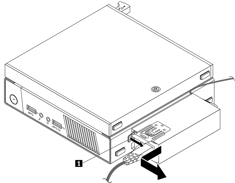
Figure 36. Retrait du système de retenue du bloc d'alimentation
