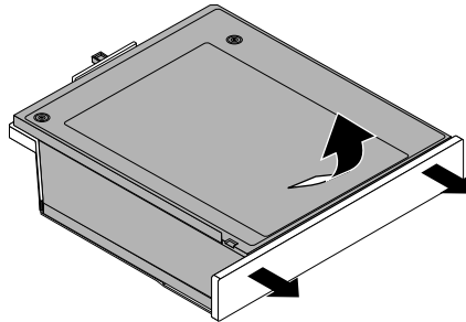
Figure 25. Retrait de la carte de l'unité de disque dur du système de retenue
