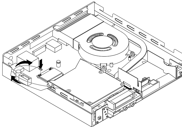
Figure 56. Branchement du câble de l'antenne Wi-Fi avant
