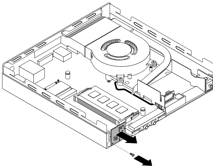
Figure 47. Retrait de la carte de l'interrupteur d'alimentation
