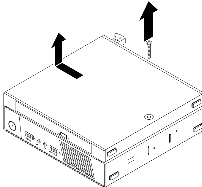
Figure 23. Retrait du coffret du disque optique
