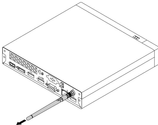
Figure 59. Retrait de l'antenne Wi-Fi arrière
