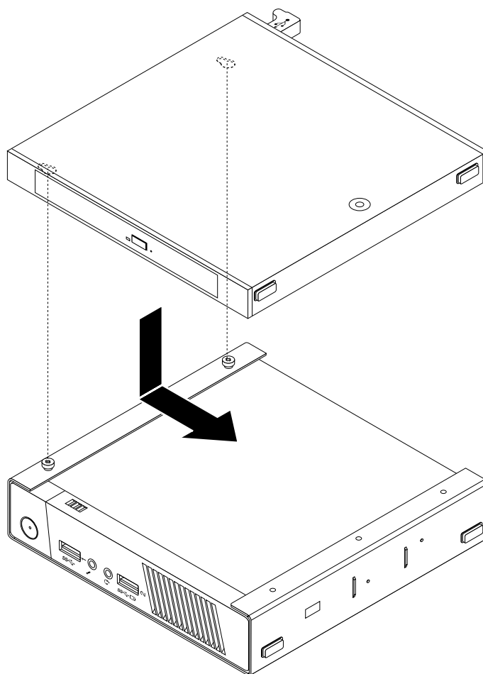
Figure 31. Installation du coffret du disque optique
