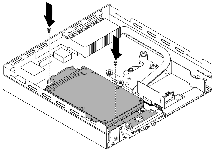
Figure 42. Installation des vis de fixation de l'unité de disque dur
