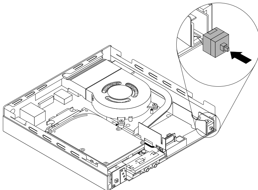
Figure 65. Installation de l'interrupteur de détection de présence du carter
