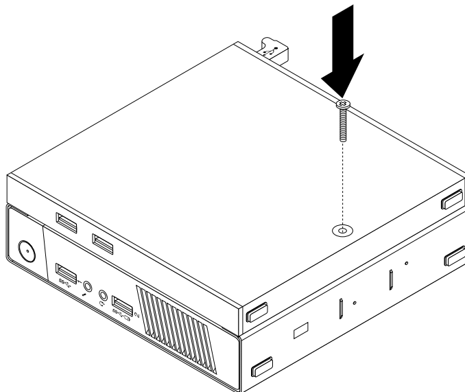
Figure 35. Installation de la vis de fixation du boîtier d'E-S
