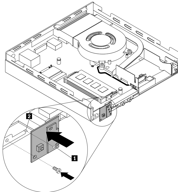
Figure 48. Installation de la carte de l'interrupteur d'alimentation
