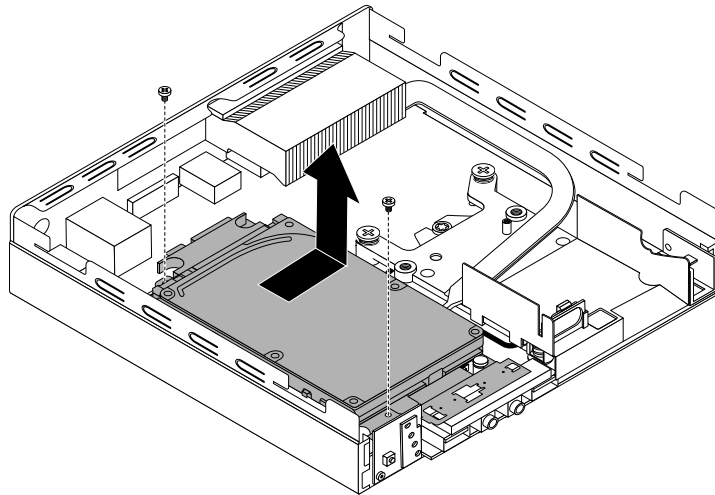
Figure 40. Retrait de l'unité de disque dur
