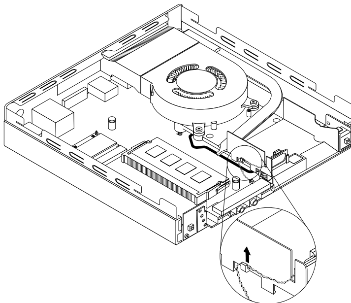
Figure 60. Dégagement du câble du haut-parleur interne
