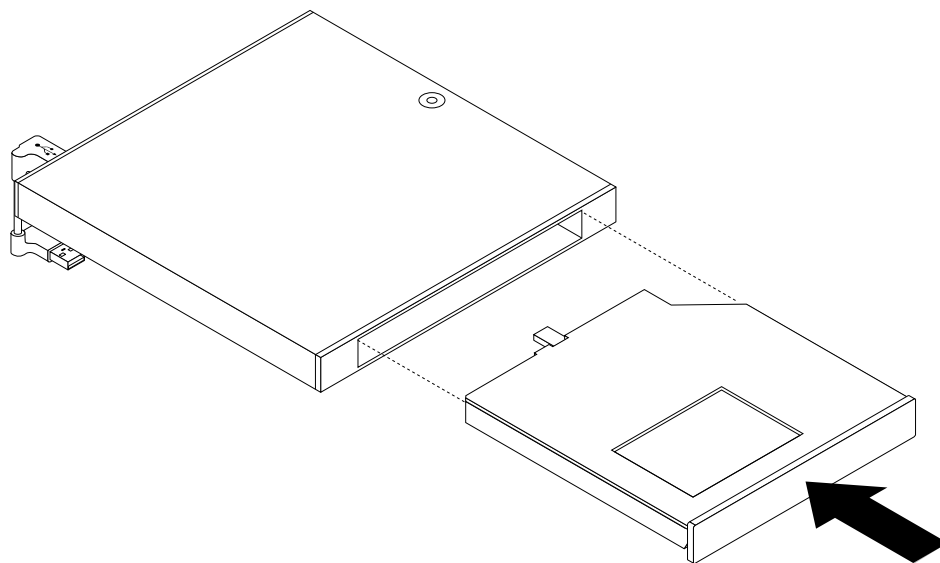
Figure 30. Installation du système de retenue dans le coffret du disque optique
