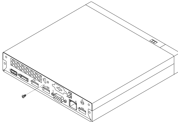
Figure 75. Installation de la vis de fixation du carter de l'ordinateur
