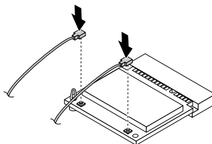
Figure 52. Branchement des câbles d'antenne Wi-Fi
