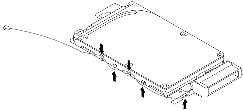
Figure 55. Acheminement du câble de l'antenne Wi-Fi avant
