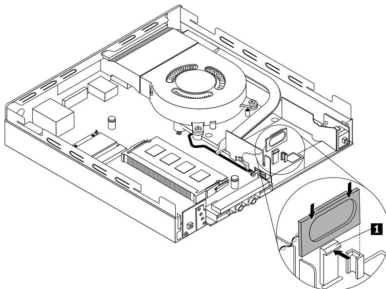
Figure 62. Installation du haut-parleur interne
