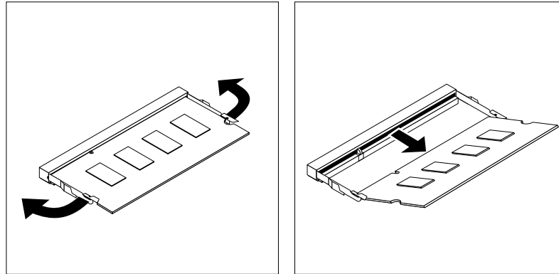
Figure 43. Retrait du module de mémoire
