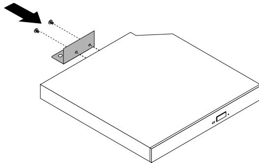
Figure 18. Installation de la plaque métallique du disque optique
