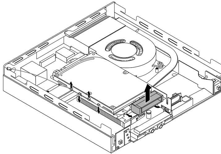
Figure 57. Retrait du câble de l'antenne Wi-Fi avant
